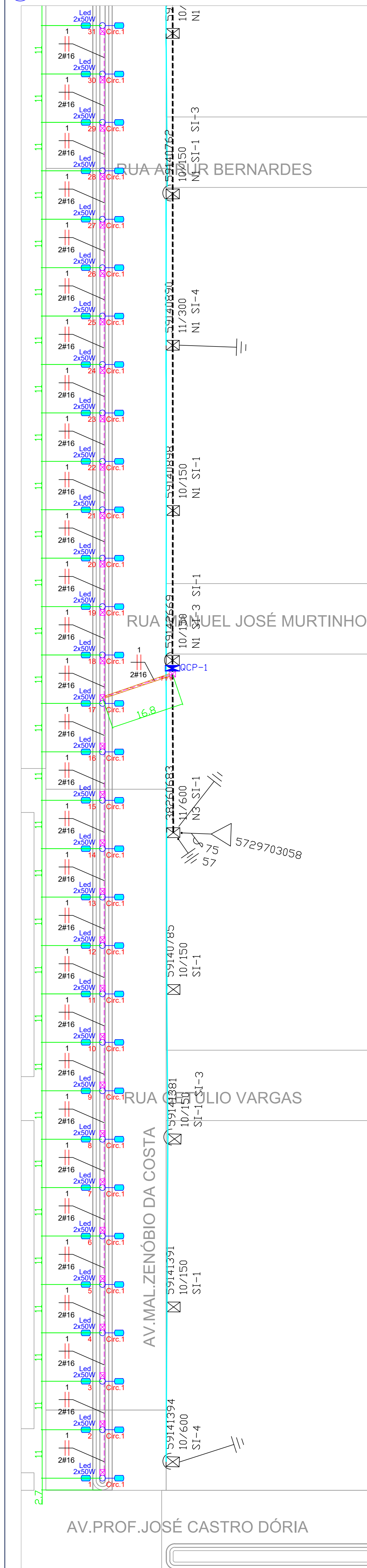
01 Proj. Elétrico AV. Mal.Zenóbio da Costa - ÁREA 01 Escala: 1:500
