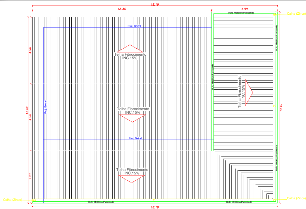
PLANTA / COBERTURA
