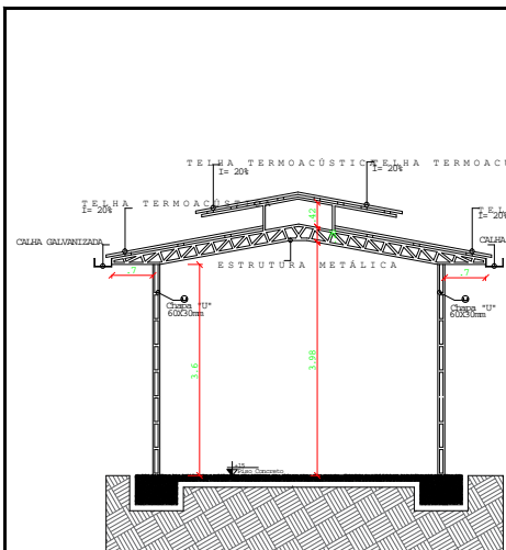
CORTE AA
