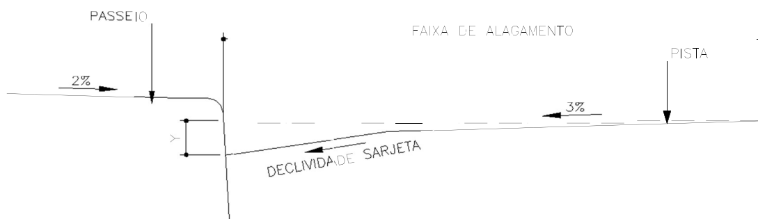
Figura da seção típica da via
