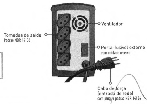
Modelo 600 VA
