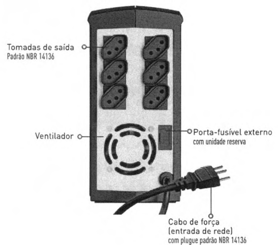
Modelo 800 VA
