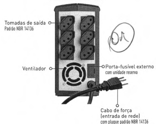
Modelo 800 VA
