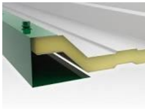
Figura 12: acabamento lateral de telha termo acustica.
