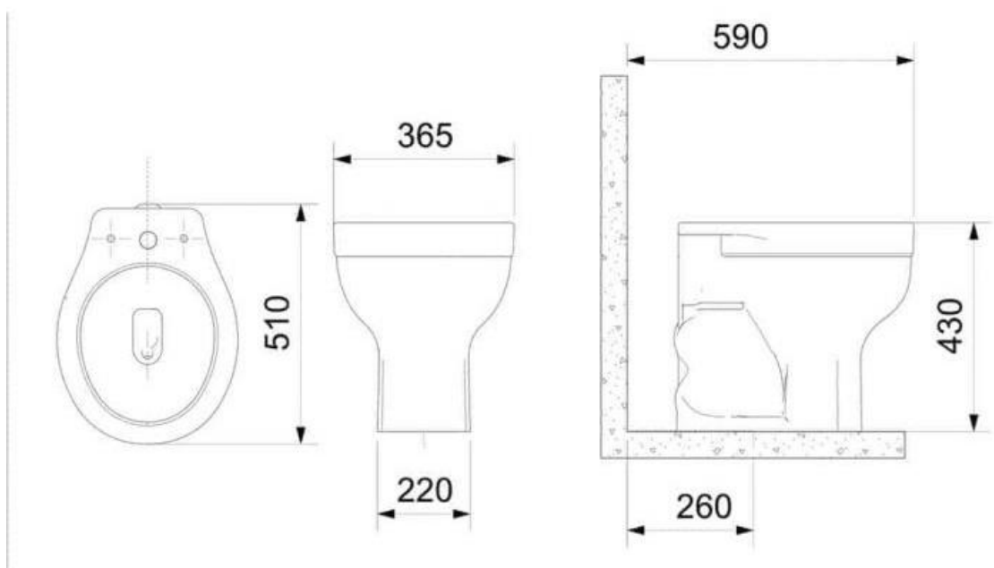
Figura 22: Detalhamento vaso PNE
