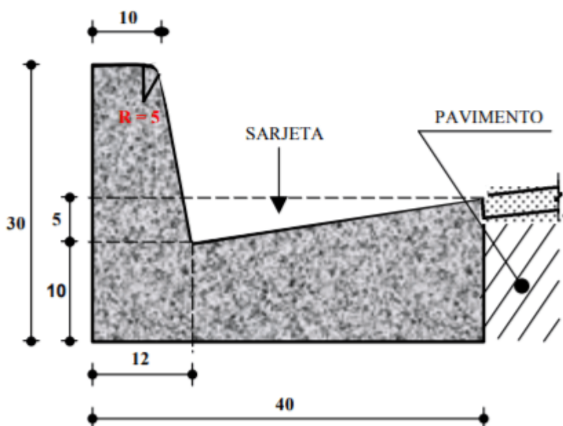
Figura 8: sarjeta e mei-fio
